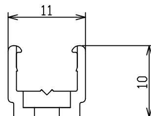
A-A'断面図
