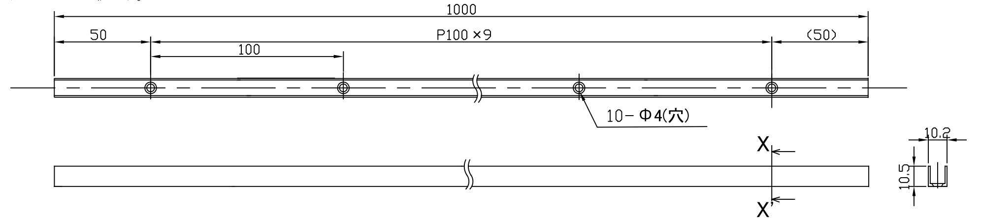
X-X'断面図
