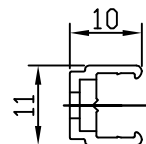
A-A' 断面図
