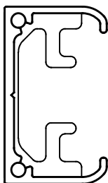
側面図 (1/1)
